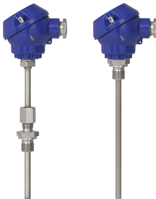
Рис. слева: Модель TC10-D с технологическим присоединением с компрессионным фитингом Рис. справа: Модель TC10-D с технологическим присоединением с шестигранной втулкой с двухзаходной резьбой
