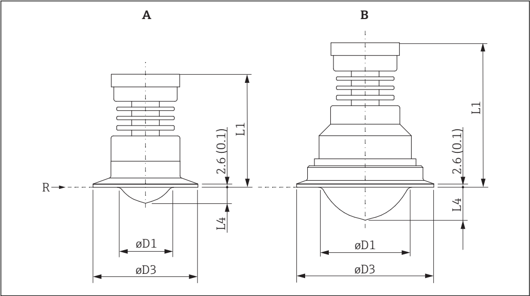
36 Размеры прибора с соединением Tri-Clamp. Единица измерения мм (дюйм)
