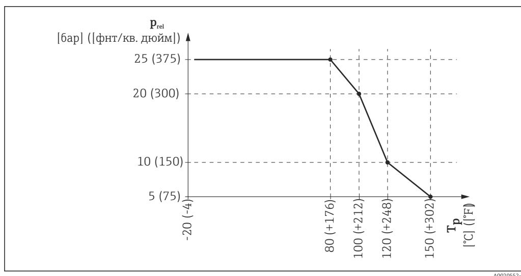
25 Прибор FMR54 с планарной антенной: допустимый диапазон рабочей температуры и рабочего давления
