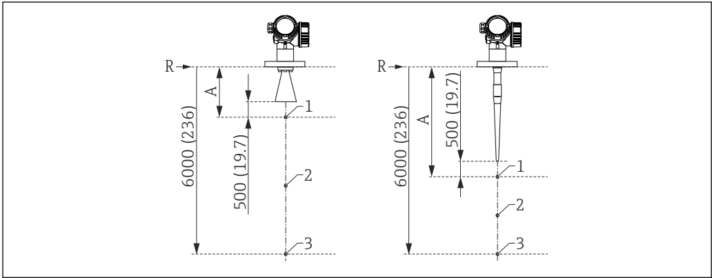
42 Точки калибровочного протокола по 3 точкам; единица измерения: мм (дюймы)
