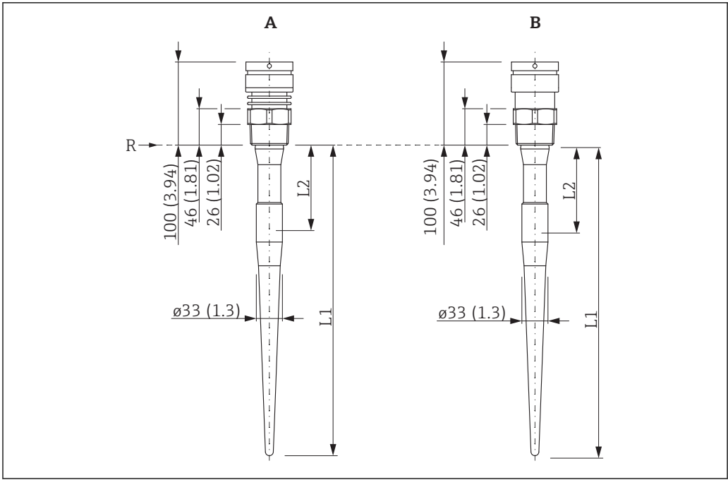
30 Размеры прибора с резьбой. Единица измерения мм (дюйм)
