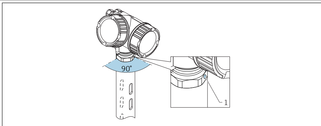
21 Монтаж в успокоительной трубе
