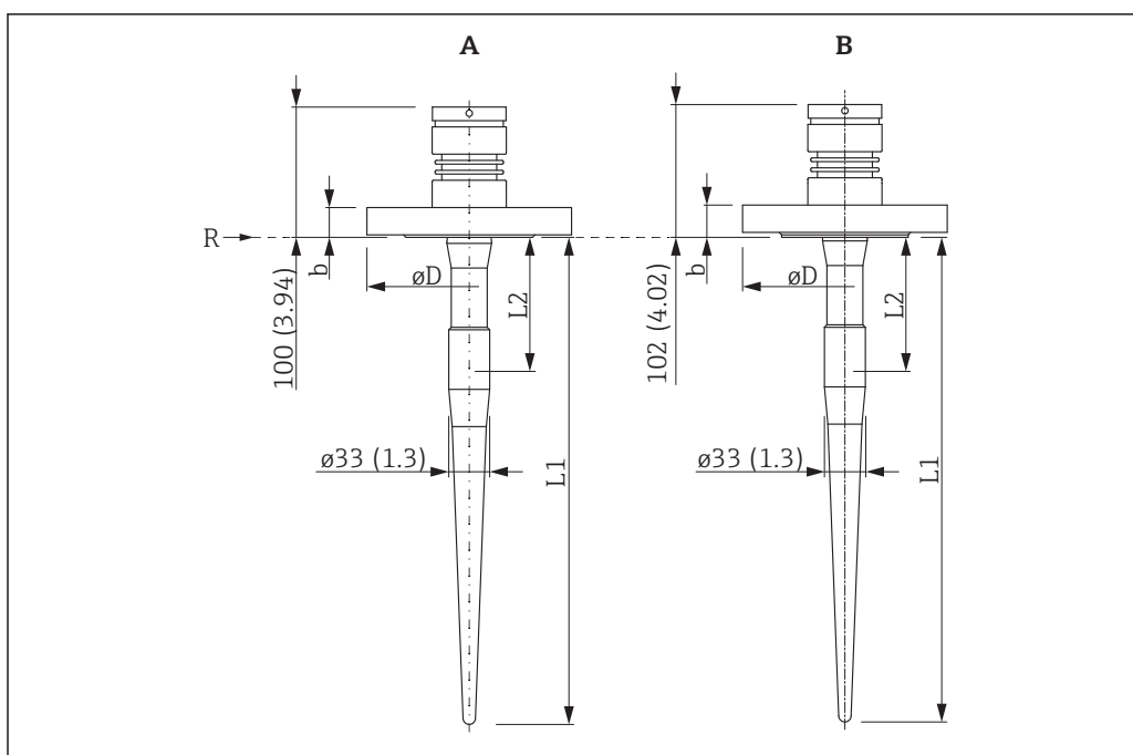
29 Размеры прибора с фланцем. Единица измерения мм (дюйм)
