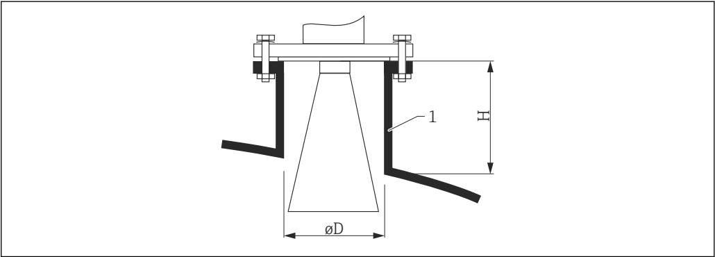
20 Высота и диаметр патрубка для рупорной антенны
