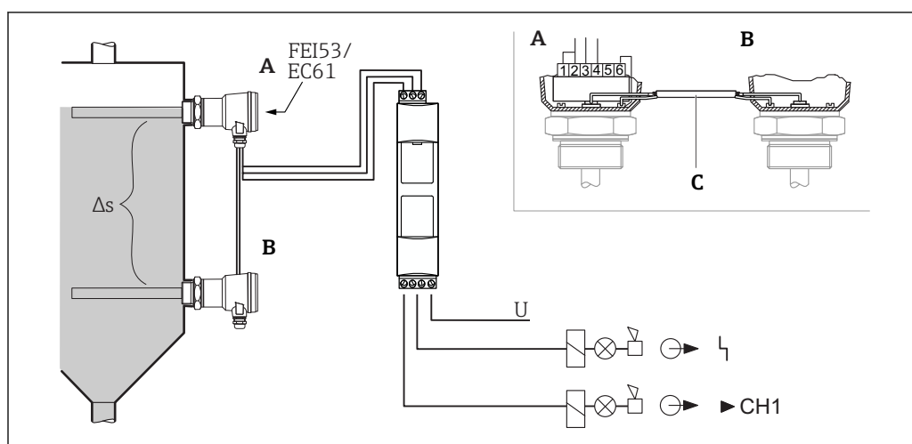
4 Двухточечный контроль с использованием двух полностью или частично изолированных зондов (A, B) и электронной вставки FEI53. Зонды соединяются коаксиальным кабелем (C).
