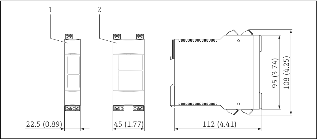
Размеры, мм (дюймы) 1 1-канальный детектор Nivotester 2 3-канальный детектор Nivotester
