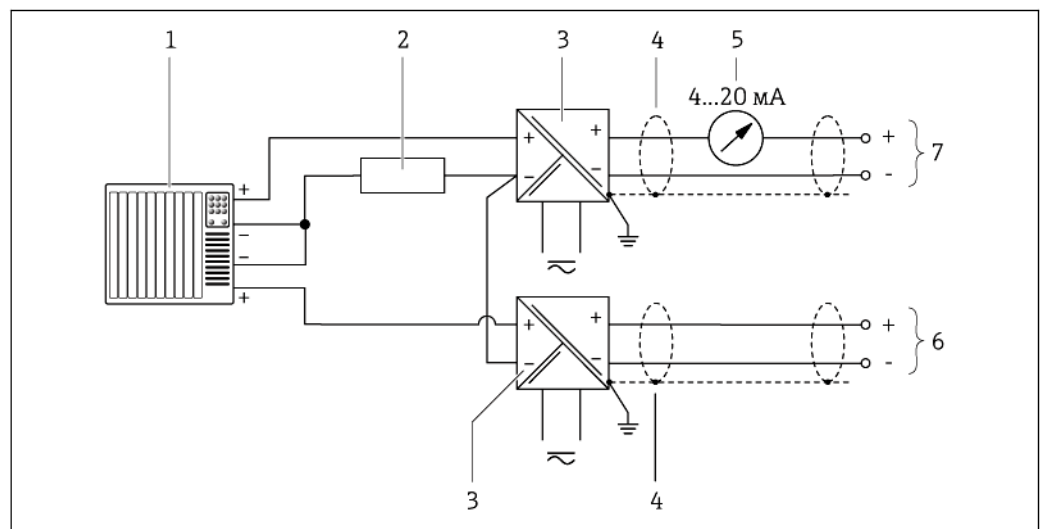
5 Пример подключения для входа HART с общим минусом
