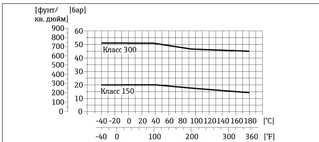
13 Материал присоединения к процессу, углеродистая сталь, A105
