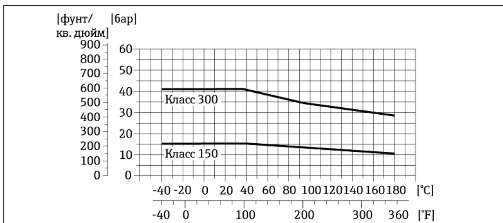
14 Материал присоединения к процессу: нержавеющая сталь, F316L
