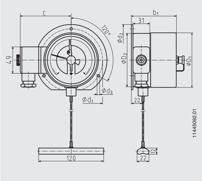
Фланец поверхностного монтажа
