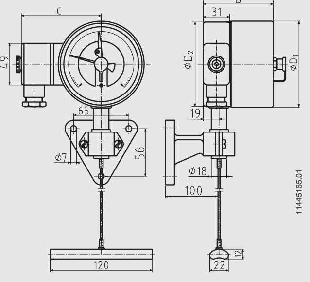
Монтажный кронштейн
