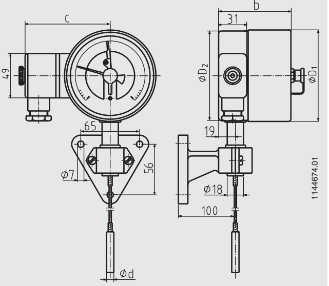
Монтажный кронштейн
