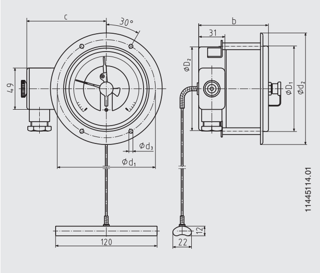
Приборы с ном. диаметром 100 с фланцем для монтажа в панель
